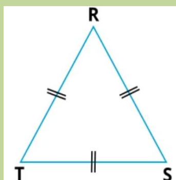
Triangle équilatéral RST
