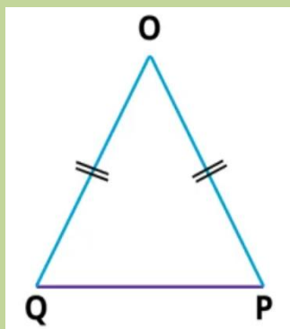
Triangle isocèle OQP
